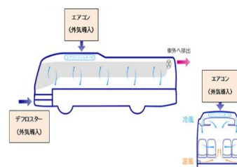
外気導入換気イメージ
